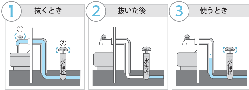
①蛇口をいっぱいに向け水を出す ②水抜き栓のハンドルを時計回りに止まるまで回す
